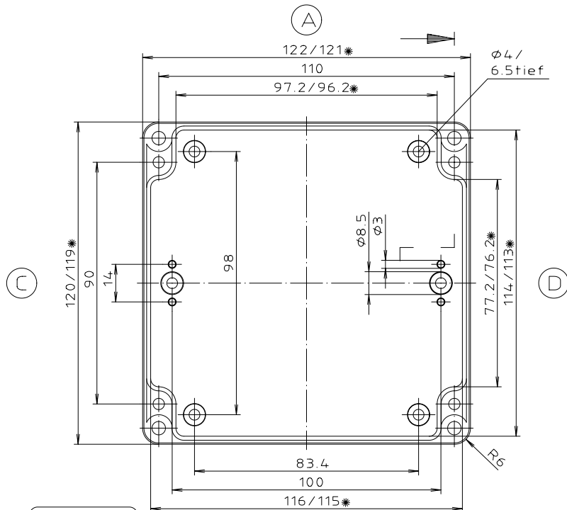
Unterteil
